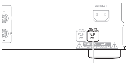
SPEAKER IMPEDANCE-Wahlschalter
